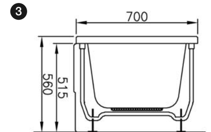
Side View Yan Görünüş
