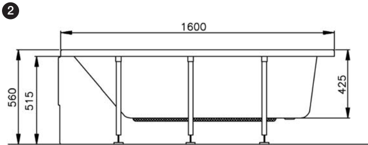
Front View Ön Görünüş
