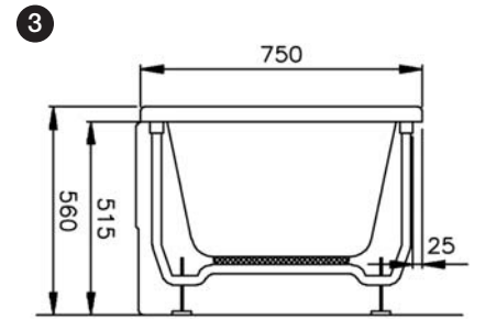
Side View Yan Görünüş
