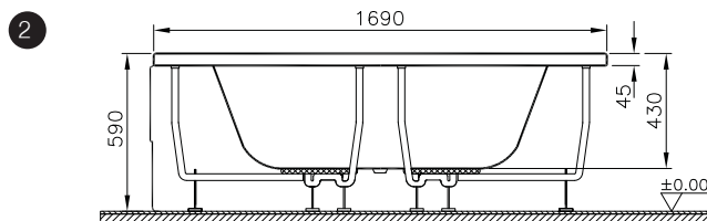
Front View Ön Görünüş
