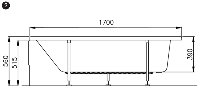
Front View Ön Görünüş
