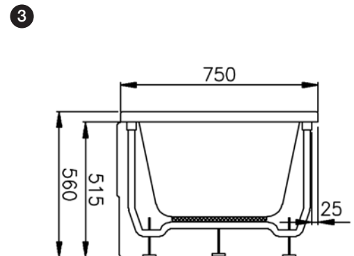
Side View Yan Görünüş
