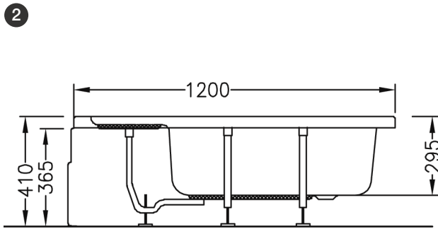
Front View Ön Görünüş
