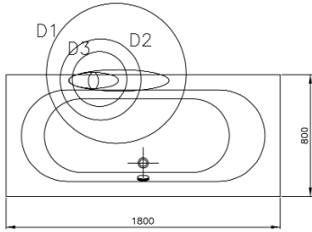
Faucet Application Places / Batarya Uygulama Yerleri
