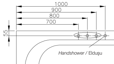
Bath Filler 4 Holes / Dört Delikli Batarya
